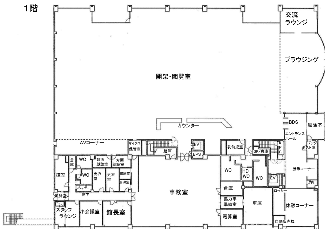
(4) 平面图
